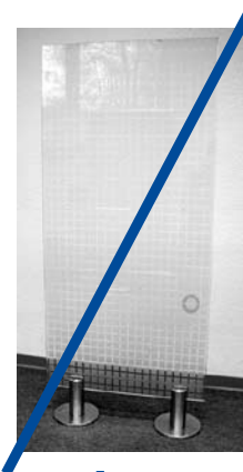
FALSCH!
